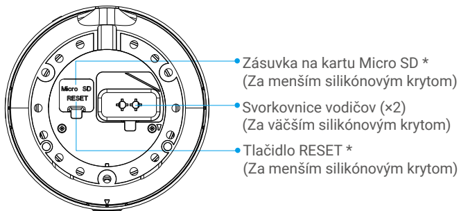
Pohľad zhora
